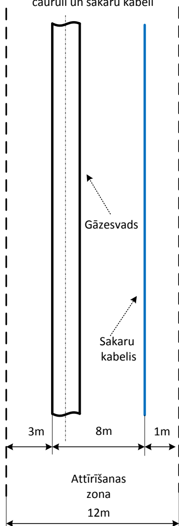
Shēma ar vienu gāzesvada cauruli un sakaru kabeli
