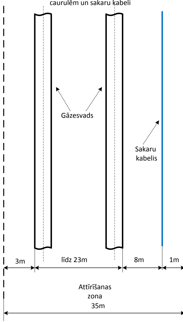
Shēma ar divām gāzesvada caurulēm un sakaru kabeli
